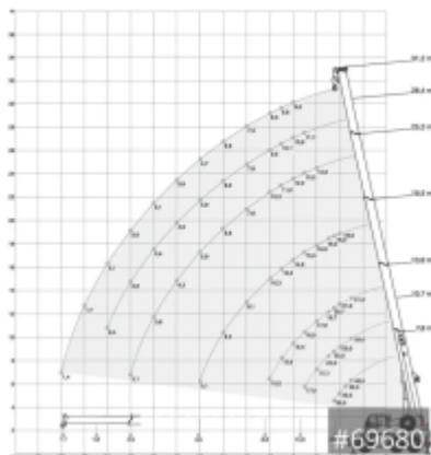
Autokran DEMAG AC 40 City
